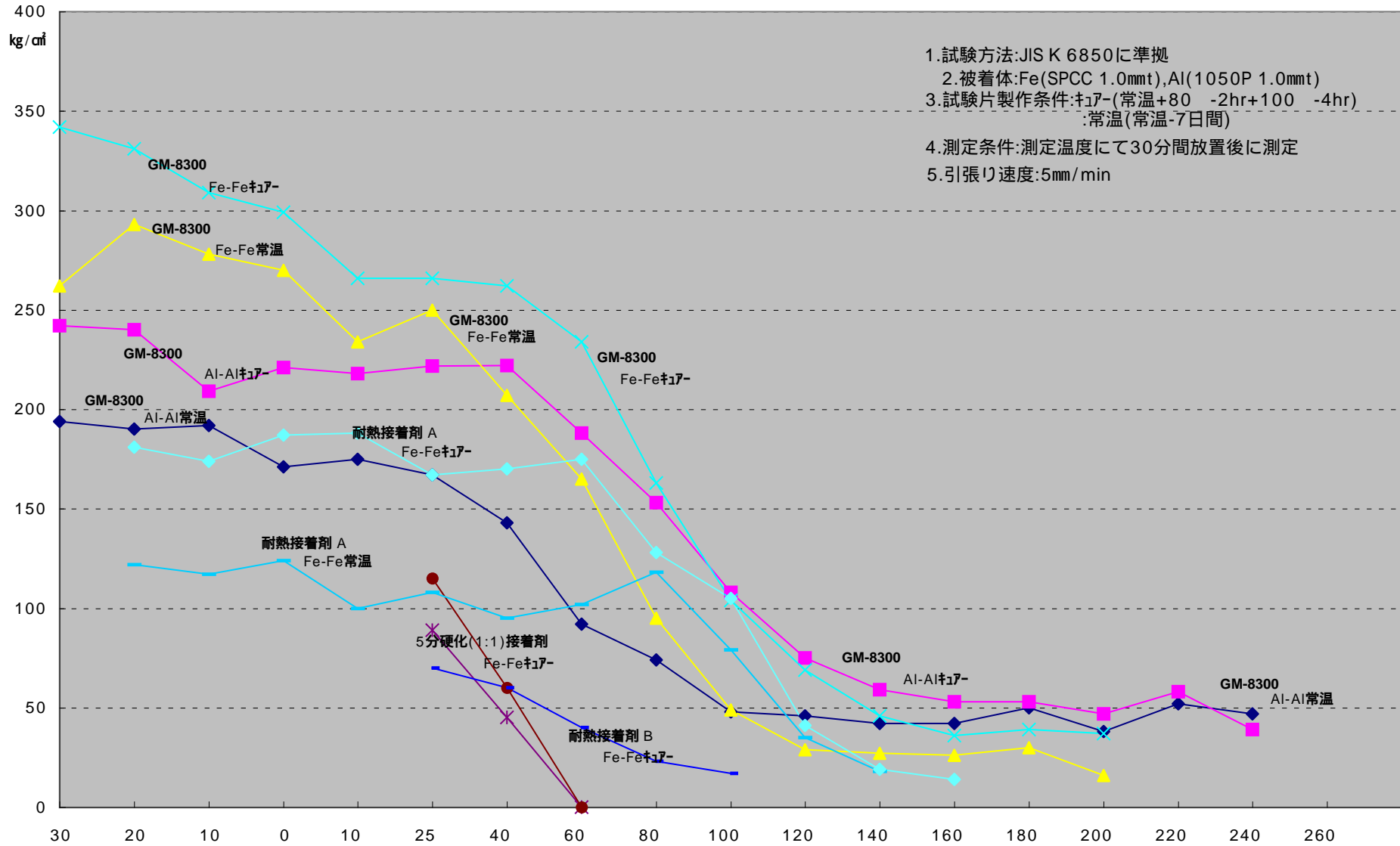
雰囲気温度と測定値の関係(引張り接着剪断強さ)
